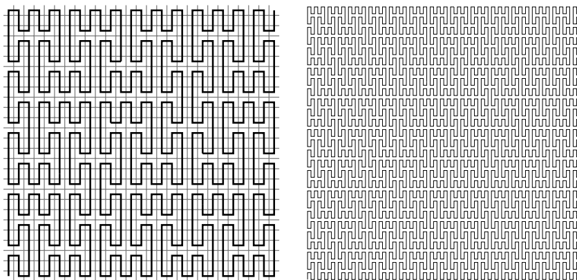
Figur 4: Tredje og fjerde tilnærming til Peano-kurven.
