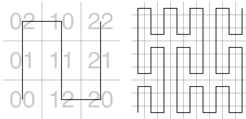
Figur 3: Første og annen tilnærming til Peano-kurven.
