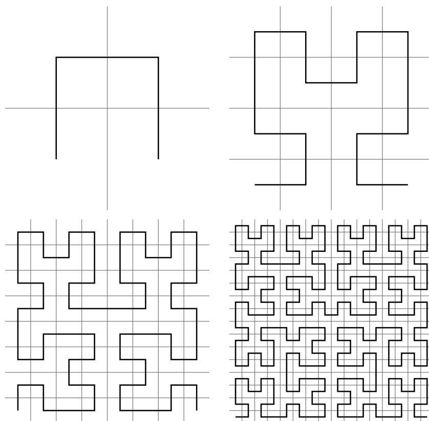
Figur 5: Første til fjerde tilnærming til Hilbert-kurven.
