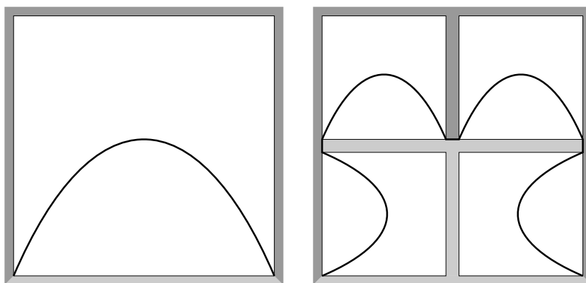
Figur 6: Nullte og første tilnærming til Hilbert-Osgood-kurven.
